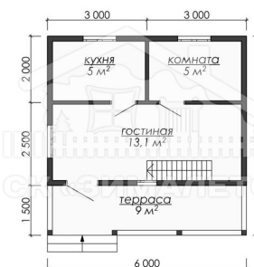
План 1-го этажа
