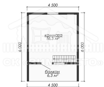
План 2-го этажа
