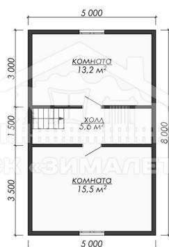
План 2-го этажа
